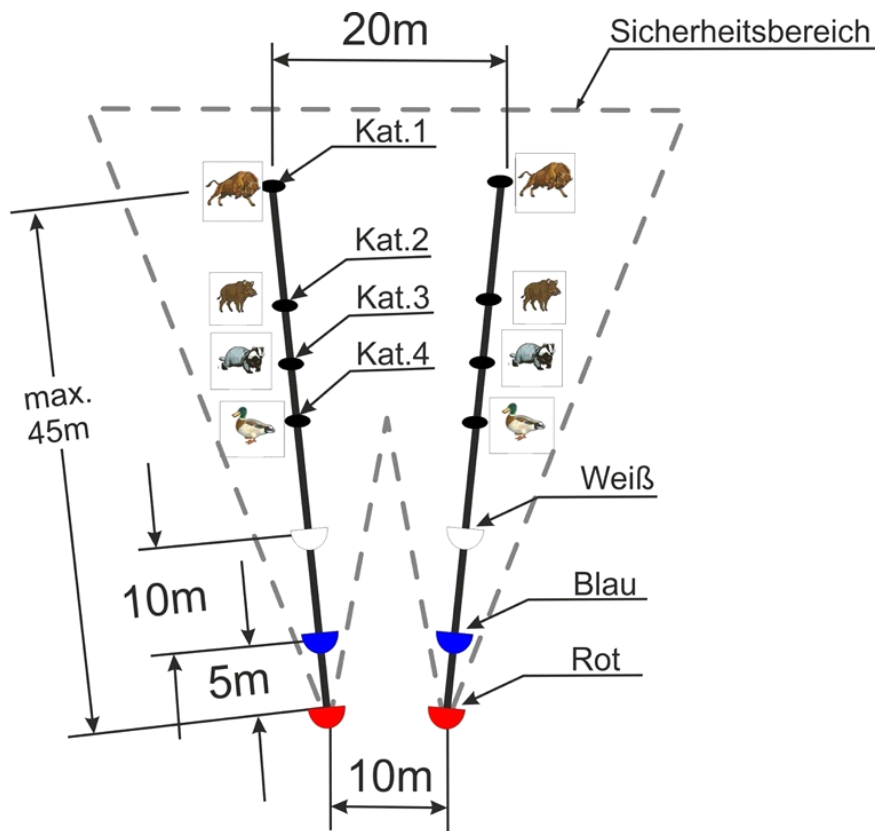
Prinzipische Skizze ohne Maßstab!
